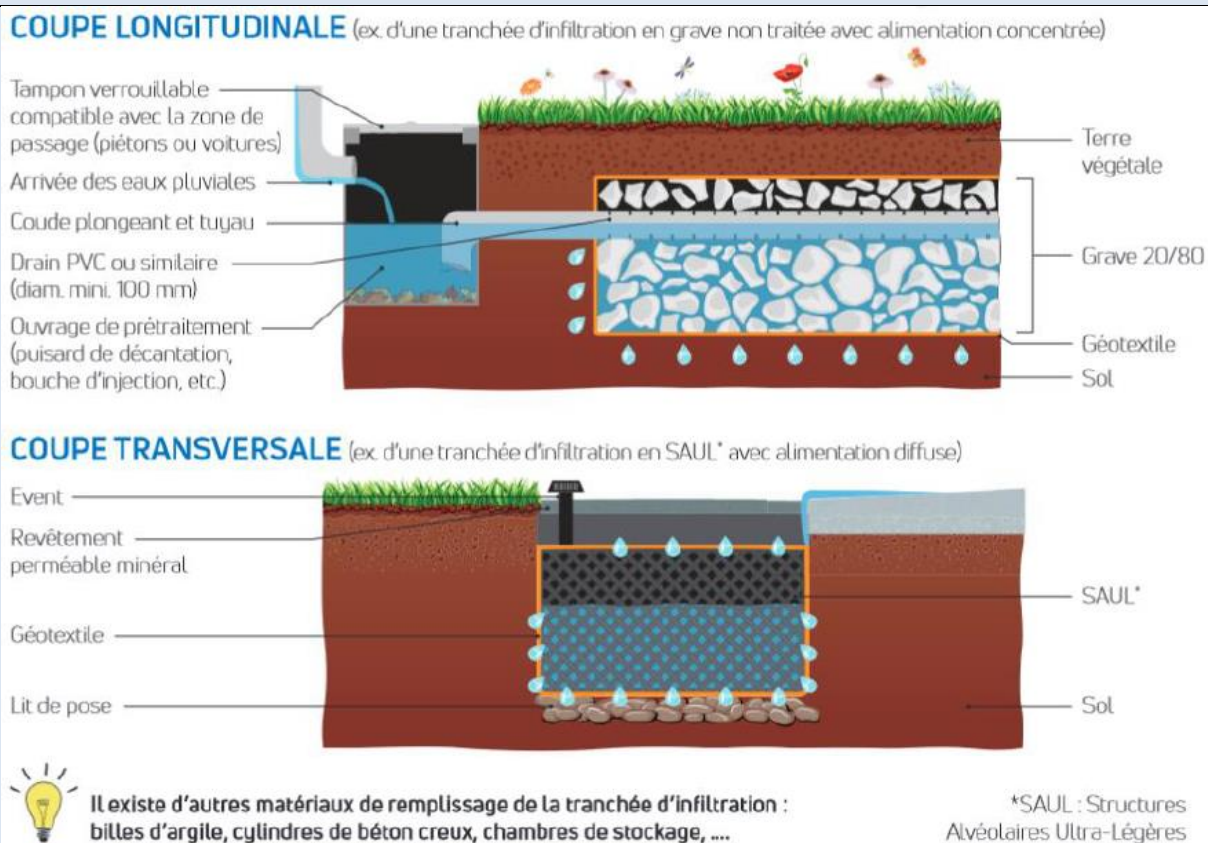
Figure 23 : Fiche technique ADOPTA d'une coupe de tranchée drainante (Source – www.adopta.fr )
